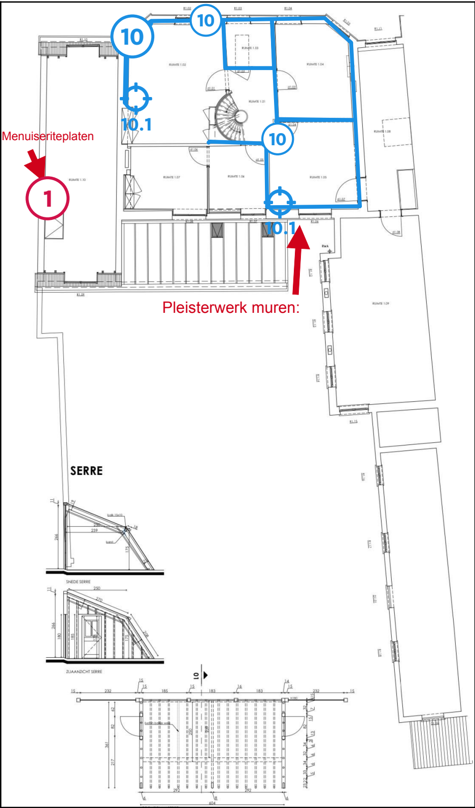
Legende van plan 1.5: Grondplan +1: pleisterwerk muren, platen zolder
