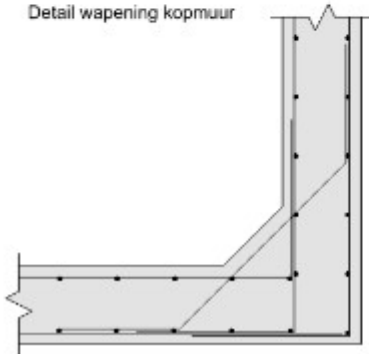
Detail wapening kopmuur
