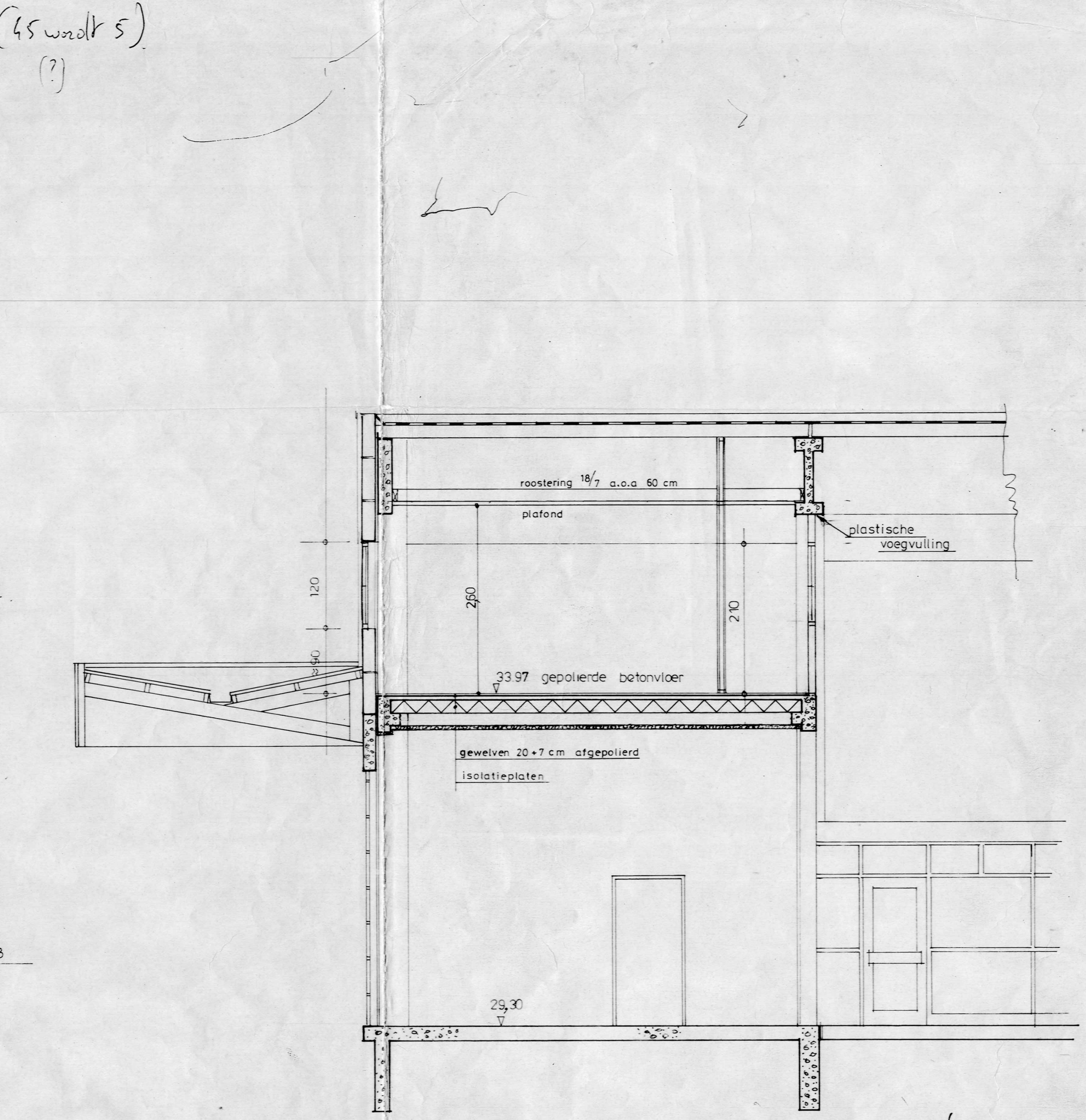
DOORSNEDE DOOR BUREEL R.T. sch. 1/50
